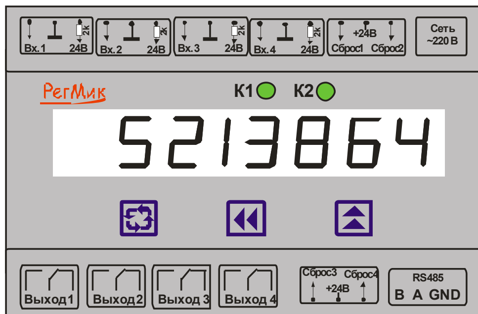
Рисунок 3.2 – Лицевая панель прибора
