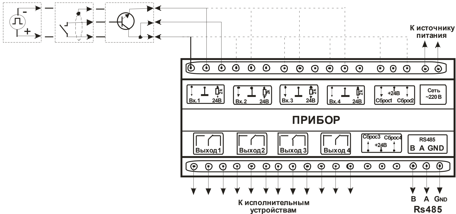
Рисунок 8.1 – Схема подключения входных датчиков, источника питания и исполнительных устройств
