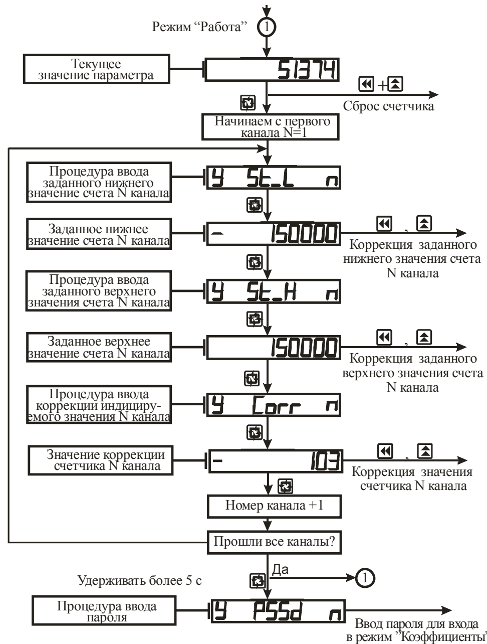
Рисунок 3.3 – Схема алгоритма работы прибора в режиме "Работа"
