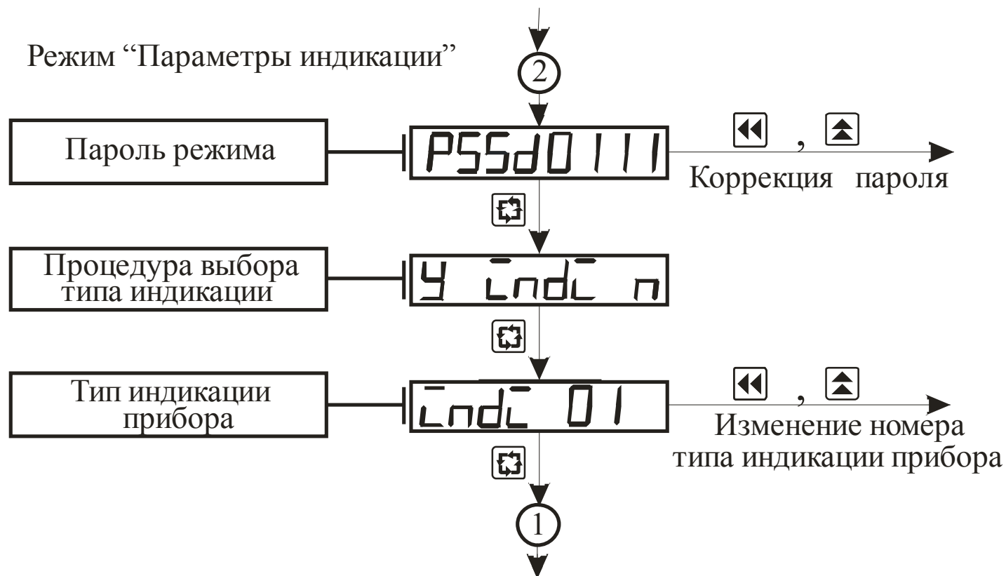
Рисунок 3.4 – Схема алгоритма работы в режиме “Параметры индикации”
